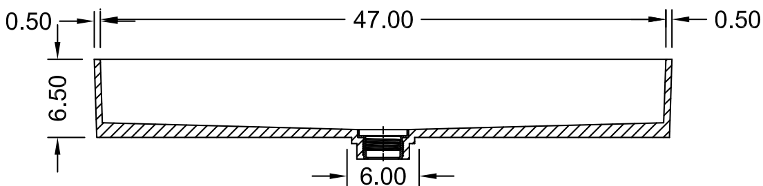
SECTION A-A
